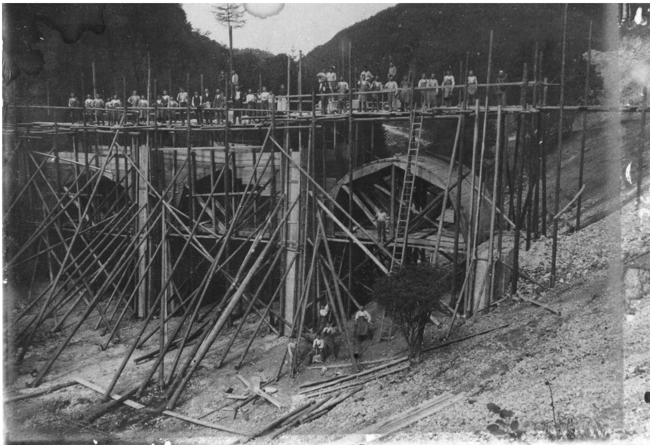
Schalungskonstruktion der Pfeiler, des Gewölbes und Fahrbahnüberbaus Bild: ca. 1906, Gemeindearchiv Blaubeuren
