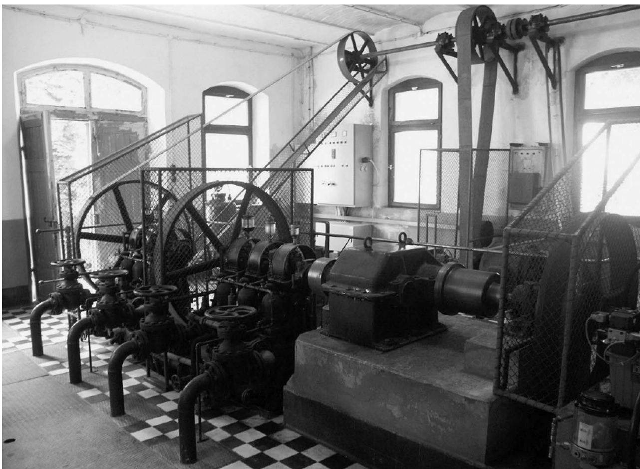
Pumpwerk (links) angetrieben von einer Francis-Turbine mit horizontaler Welle (rechts) der Fa. Voith, 1935 Bild: Gemeindearchiv
