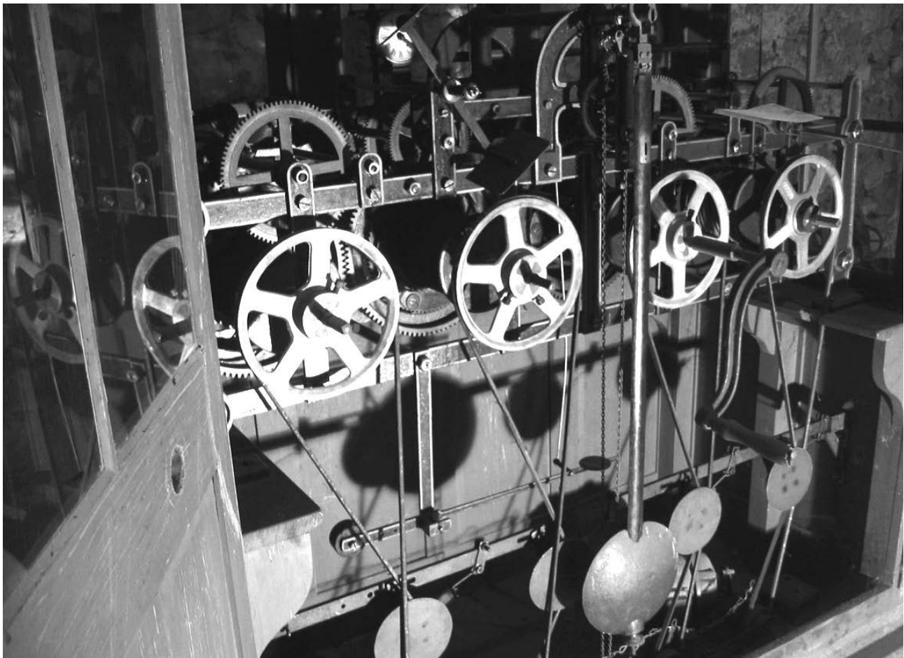
Turmuhrwerk 300 D, eingebaut 1921 von der Firma Hörz in Ulm. Bild: Wolfgang Schlenk
